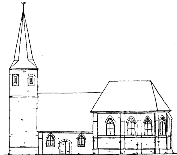
SEITENANSICHT
