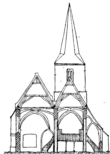
QUERSCHNITT
